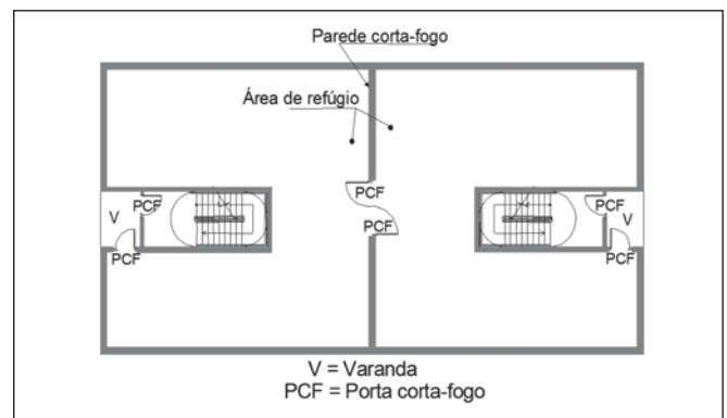
Figura 17: Desenho esquemático da área de refúgio
